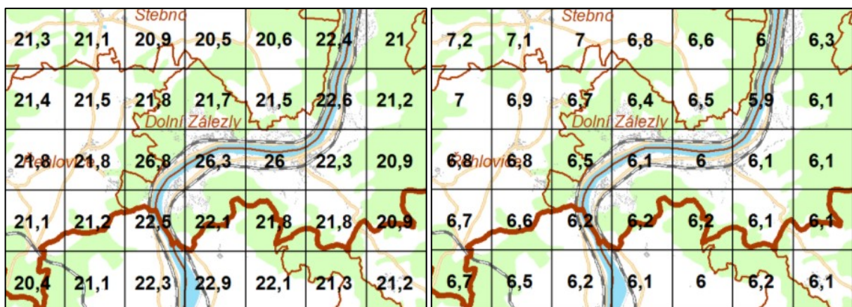
Obr. 7 Koncentrace PM 10 (vlevo) a SO 2 (vpravo) v okolí Dolních Zálezel (2014-2018) zdroj: www.portal.chmi.cz
